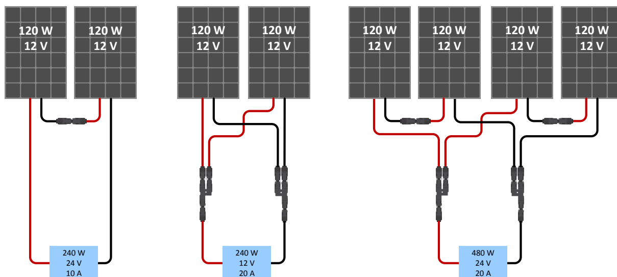
Voorbeelden van serie-, parallele- en serie / parallel zonnepanelen.
