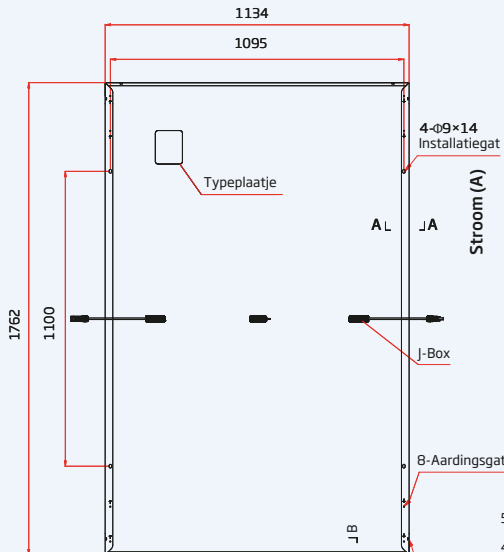
Achteraanzicht
