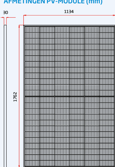
Vooraanzicht
