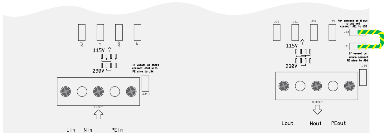
AC-uitgang nul (N) naar aardingskoppeling (PE)
